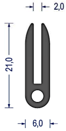
Artikel-Nr. 0202 EPDM · 45° ShoreA · schwarz VE: Bund á 100m
