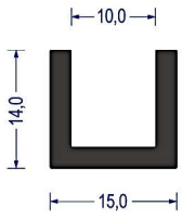
Artikel-Nr. 1009 EPDM · 65° ShA · schw. VE: Bund á 50m
