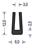
Artikel-Nr. 0319 EPDM · 60° ShA · schw. VE: Bunde á 100m
