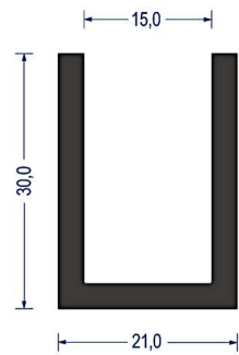
Artikel-Nr. 1504 EPDM · 65° ShoreA · schwarz VE: Bund á 25m
