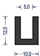
Artikel-Nr. 0502 EPDM · 60° ShA · schw. VE: Bund á 100m
