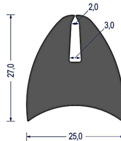
Artikel-Nr. 0298 EPDM · 55° ShoreA · schwarz VE: Bund á 25m
