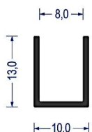
Artikel-Nr. 0817 EPDM · 65° ShA · schw. VE: Bund á 100m
