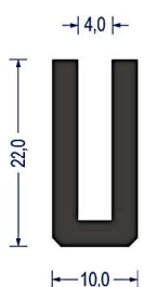
Artikel-Nr. 0405 CR · 50° ShA · schwarz VE: Bund á 25m
