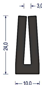
Artikel-Nr. 0367 EPDM · 65° ShA · schw. VE: Bund á 15m rundgeheizt, talkumiert
