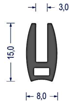
Artikel-Nr. 0366 EPDM · 65° ShoreA · schwarz VE: Bund á 50m
