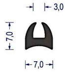
Artikel-Nr. 0308 EPDM · 50° ShoreA schwarz VE: Bund á 200m
