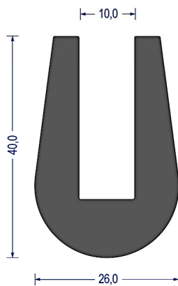
Artikel-Nr. 1065 EPDM · 65° ShoreA · schwarz VE: Bund á 25m
