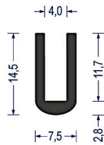
Artikel-Nr. 0464 EPDM · 60° ShoreA schwarz VE: Bund á 100m
