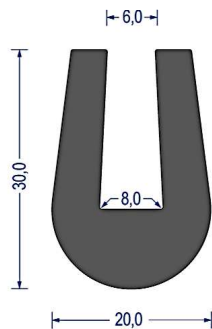
Artikel-Nr. 0855 EPDM · 65° ShoreA · schwarz VE: Bund á 25m
