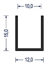
Artikel-Nr. 1022 EPDM · 65° ShA · schw. VE: Bund á 50m
