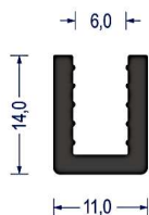
Artikel-Nr. 0601 PVC · 70° ShA · schw. VE: Bund á 100m
