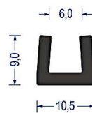
Artikel-Nr. 0604 EPDM · 65° ShA · schw. VE: Bund á 50m
