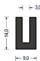
Artikel-Nr. 0339 EPDM · 65° ShA · schw. VE: Bund á 50m
