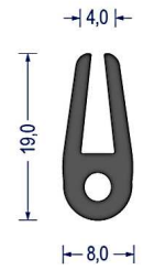
Artikel-Nr. 0472 EPDM · 65° ShoreA · schwarz VE: Bund á 50m
