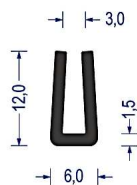
Artikel-Nr. 0318 EPDM · 60° ShA · schw. VE: Bunde á 100m
