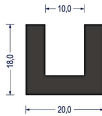
Artikel-Nr. 1003 EPDM · 65° ShoreA · schwarz VE: Bund á 30m
