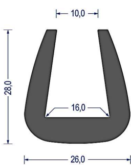
Artikel-Nr. 1602 EPDM · 85° ShoreA · schwarz VE: Bund á 25m
