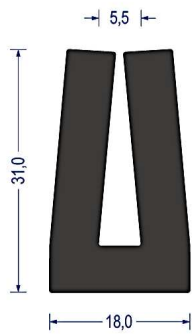
Artikel-Nr. 0593 EPDM · 65° ShoreA · schwarz VE: Bund á 15m rundgeheizt, talkumiert
