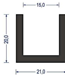
Artikel-Nr. 1502 EPDM · 65° ShoreA · schwarz VE: Bund á 25m
