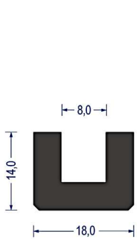
Artikel-Nr. 0805 SBR · 60° ShoreA · schwarz VE: Bund á 35m
