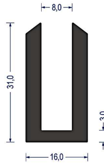
Artikel-Nr. 0801 EPDM · 65° ShoreA · schwarz VE: Bund á 25m
