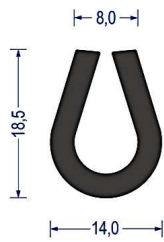
Artikel-Nr. 0809 EPDM · 70° ShoreA schwarz VE: Bund á 50m
