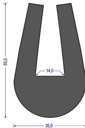
Artikel-Nr. 1401 EPDM · 65° ShoreA · schwarz VE: Bund á 25m
