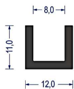
Artikel-Nr. 0803 EPDM · 65° ShA · schw. VE: Bund á 50m
