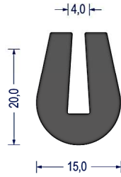
Artikel-Nr. 0488 EPDM · 65° ShoreA · schwarz VE: Bund á 50m
