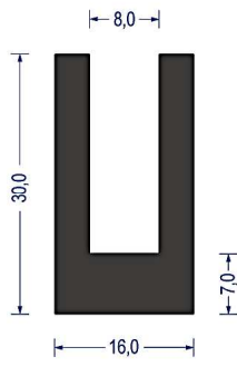
Artikel-Nr. 0802 EPDM · 65° ShoreA · schwarz VE: Bund á 25m
