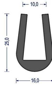
Artikel-Nr. 1002 EPDM · 45° ShoreA · schwarz VE: Bund á 50m
