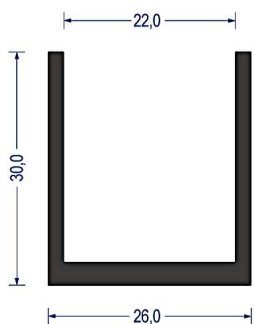
Artikel-Nr. 1603 EPDM · 65° ShoreA · schwarz VE: Bund á 25m
