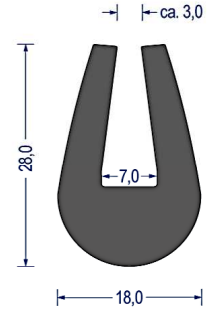
Artikel-Nr. 0702 EPDM · 70° ShoreA · schwarz VE: Bund á 25m
