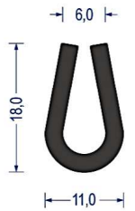
Artikel-Nr. 0601 EPDM · 60° ShoreA schwarz VE: Bund á 100m
