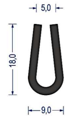
Artikel-Nr. 0503 EPDM · 65° ShoreA schwarz VE: Bund á 100m
