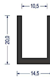
Artikel-Nr. 1075 EPDM · 65° ShA · schwarz VE: Bund á 50m
