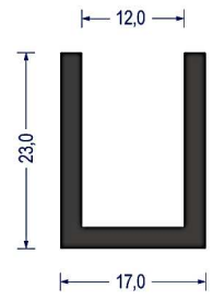
Artikel-Nr. 1204 EPDM · 65° ShoreA · schwarz VE: Bund á 50m
