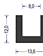
Artikel-Nr. 0804 CR · 45° ShA · schwarz VE: Bund á 40m
