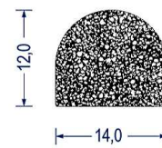
Artikel-Nr. 6121 EPDM · grau VE: Bund á 50m
