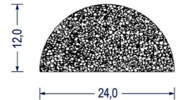
Artikel-Nr. 5972 EPDM · schwarz VE: Bund á 50m
