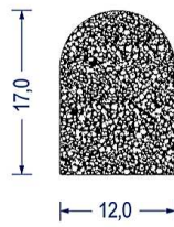
Artikel-Nr. 5618 EPDM · grau VE: Bund á 50m
