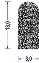
Artikel-Nr. 7632 EPDM · schwarz VE: Bund á 50m
