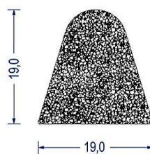
Artikel-Nr. 8372 EPDM · schwarz VE: Bund á 25m
