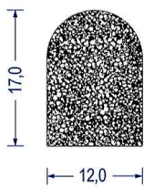
Artikel-Nr. 5618 EPDM · schwarz VE: Bund á 50m
